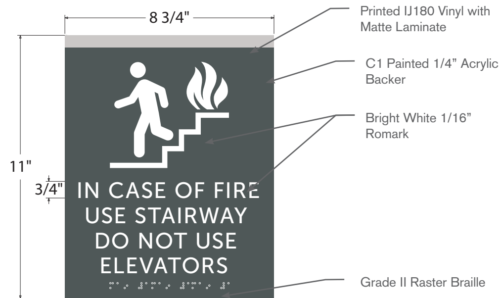
1 FRONT ELEVATION M.01 Scale: 6" = 1'
